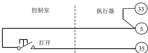
图 4-7 两线控制，有信号开，无信号关
