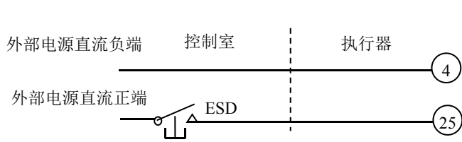
图 4-12 ESD 控制，外部供电。
