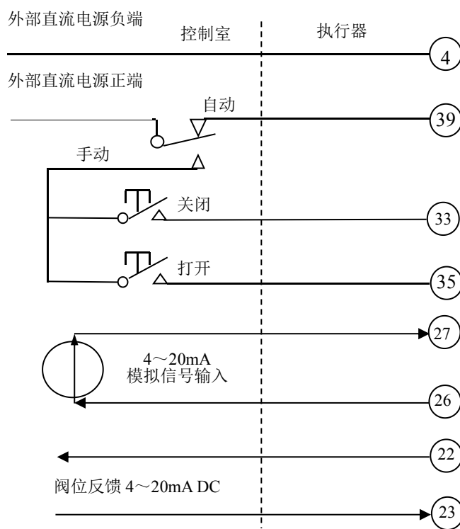
图 4-14 外部交流远方自动与手动控制及其切换电路接线图 (切换电路为外部直流电压供电)
