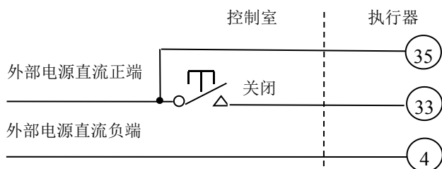
图 4-10 外部直流两线控制，有信号关，无信号开
