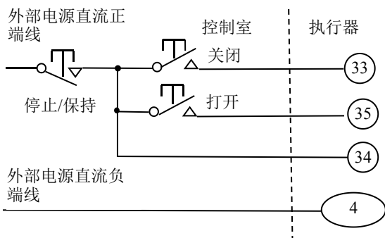
图 4-6 外部直流保持式打开、关闭、停止控制
