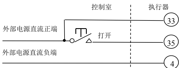
图 4-9 外部直流两线控制，有信号开，无信号关
