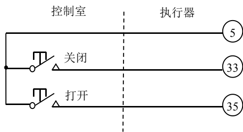
图 4-1 点动式打开/关闭控制，执行器可以停在中途任意位置
