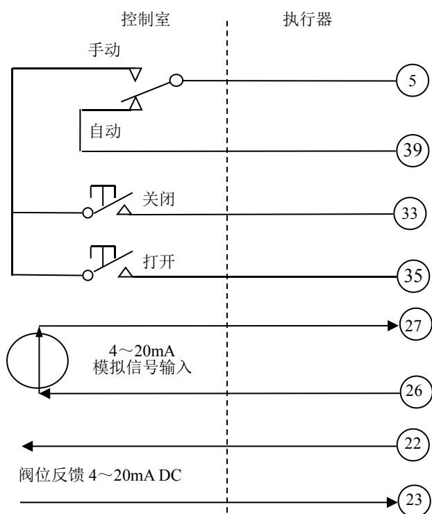
图 4-13 远方自动与手动控制及其切换电路接线图 (切换电路为内部 24V 供电)
