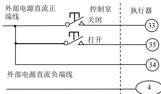
图 4-5 外部直流保持式打开 / 关闭控制，行程可逆，但不能停在中途位置
