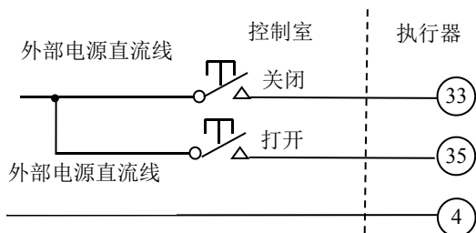
图 4-4 外部直流点动式打开/关闭控制，电动执行器可以停在中途任意位
