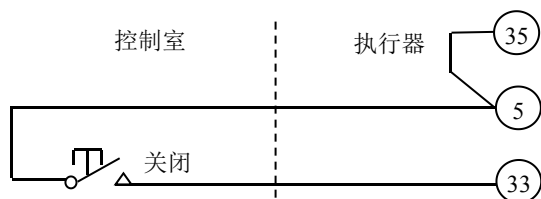
图 4-8 两线控制，有信号关，无信号开
